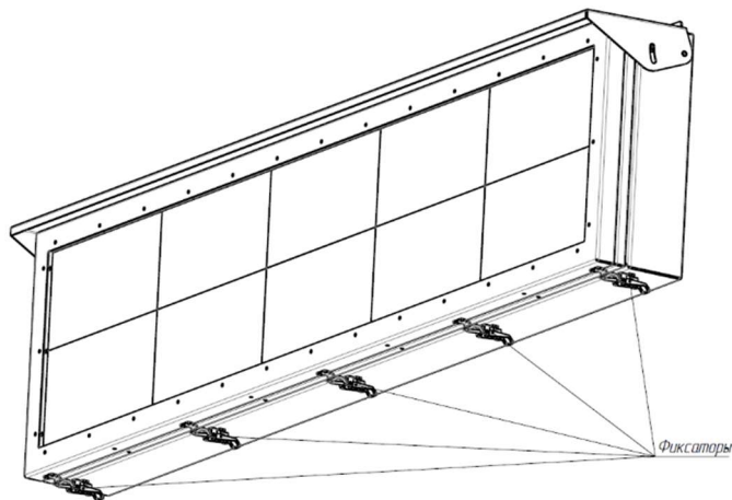
Расположение фиксаторов
