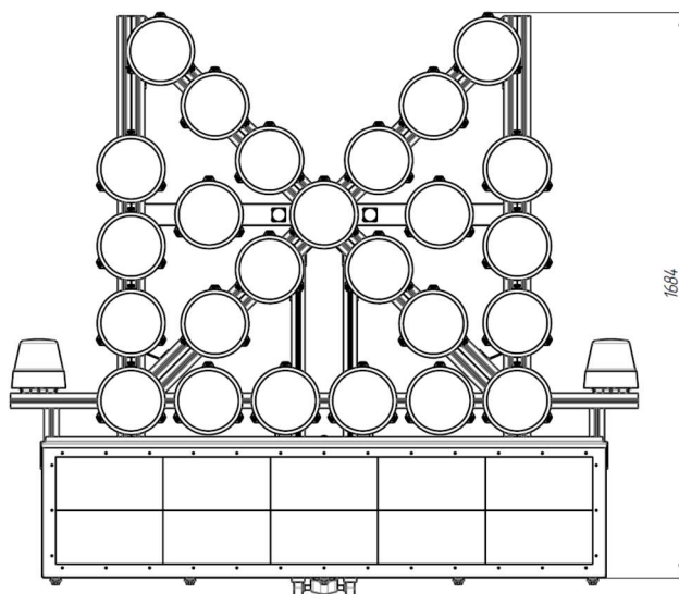
Внешний вид динамического знака аварийных работ
