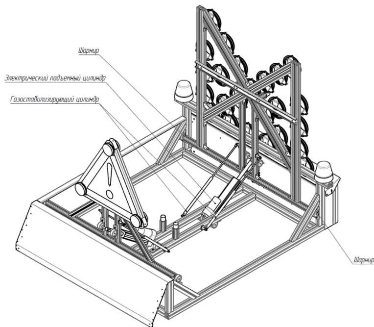
Вид на приводы подъемных элементов
