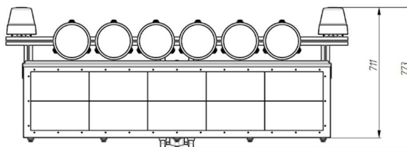
Внешний вид табло и проблесковых маяков
