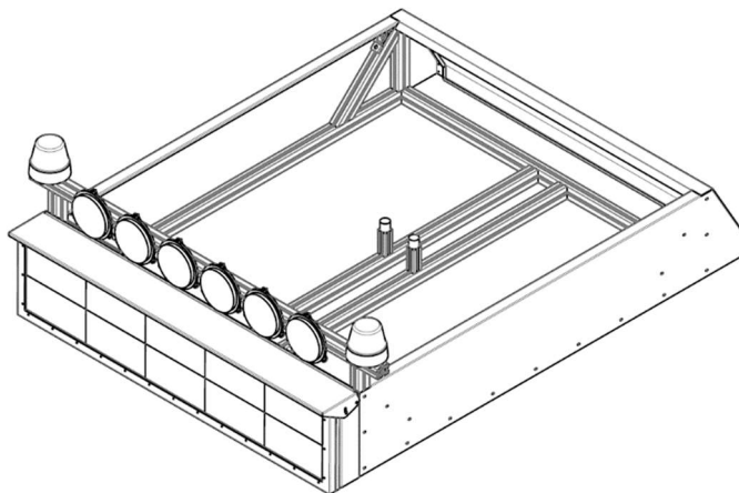
Внешний вид шасси без установленных подъемных элементов
